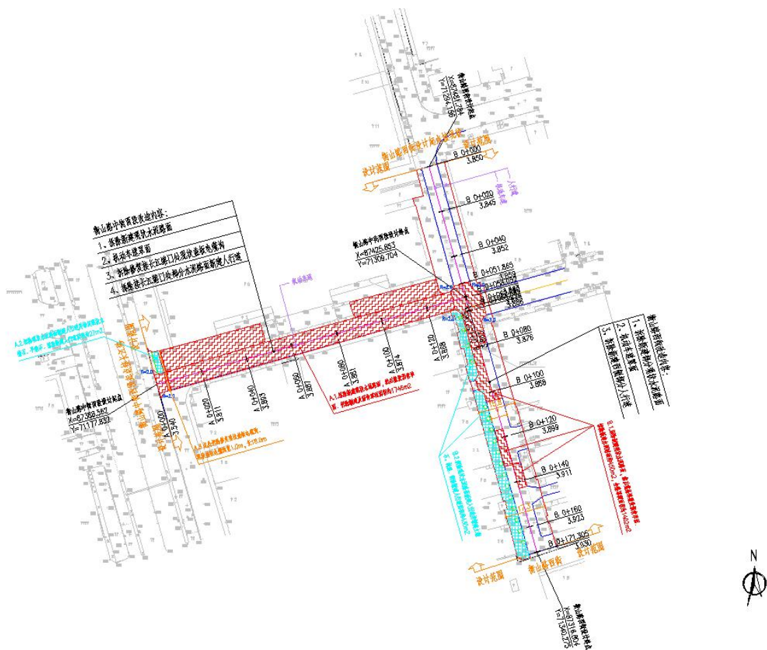
图 7-10 衡山路中街、衡山西街道路平面设计图
