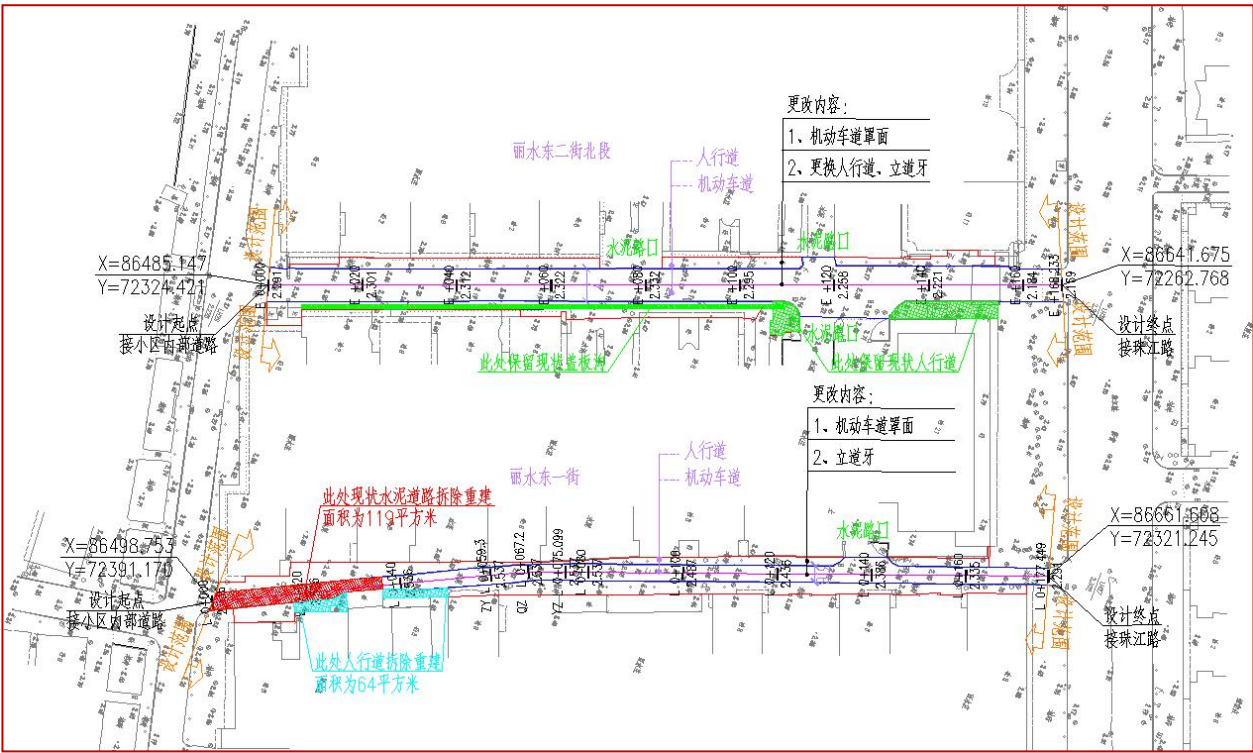
图 7-11 丽水东一、二街平面布置图
