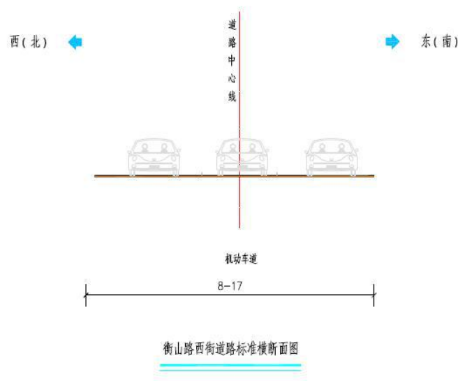
图 7-16 衡山路西街横断面图
