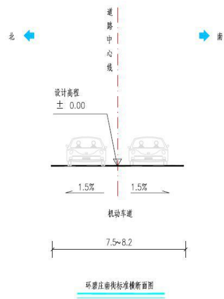
图 7-14 环碧庄南街横断面图
