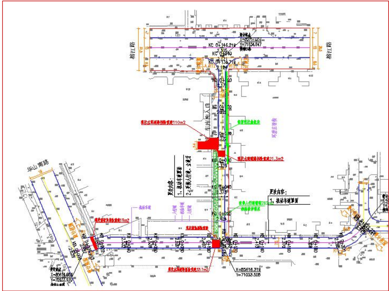
图 7-9 环碧西街、环碧南街道路平面设计图
