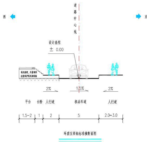
图 7-13 环碧庄西街横断面图
