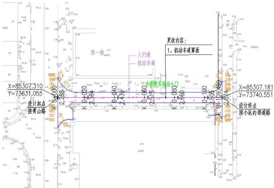
图 7-12 西一街平面布置图
