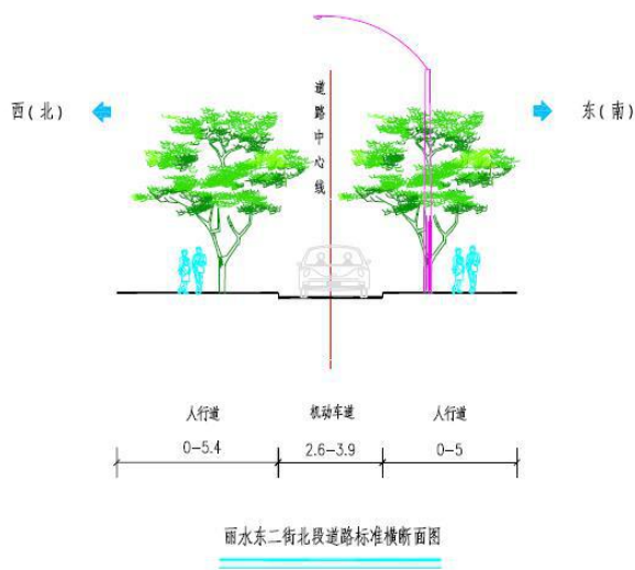
图 7-17 丽水东二街横断面图
