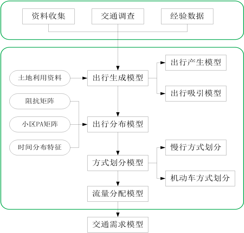
图 5-2 交通需求模型框架
