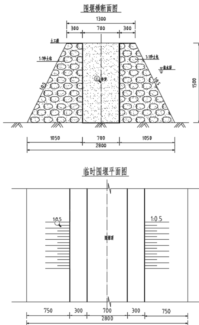
图 5-7 临时围堰
