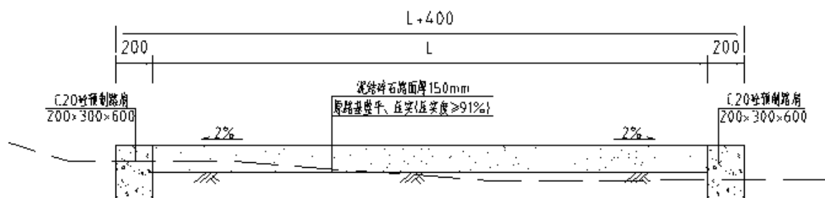
图 5-4 田间道路典型断面图 1
