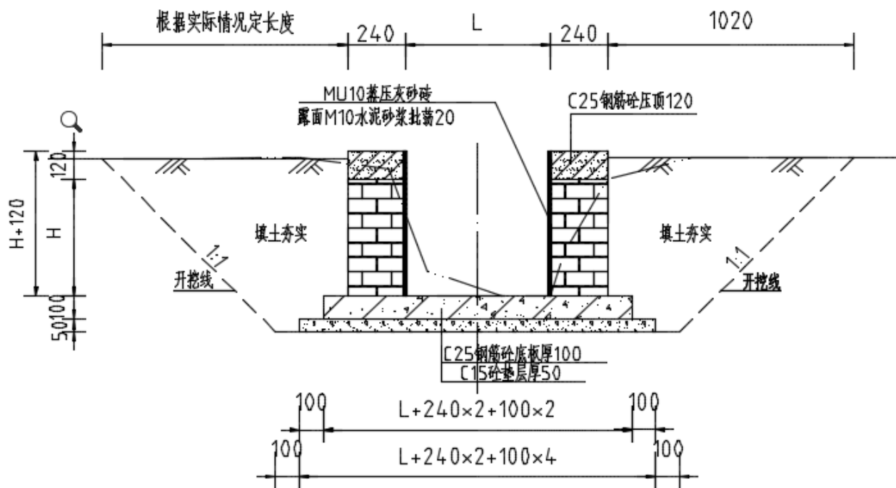
图 5-1 砖砌矩形渠道典型断面图
