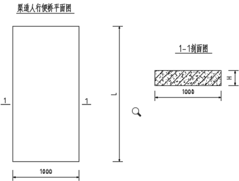
图 5-6 渠道人行便桥典型图
