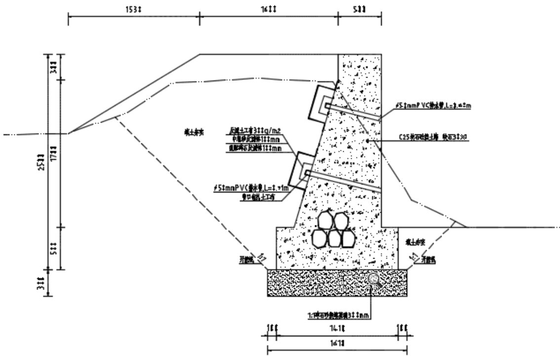
图 5-6 护岸典型断面图
