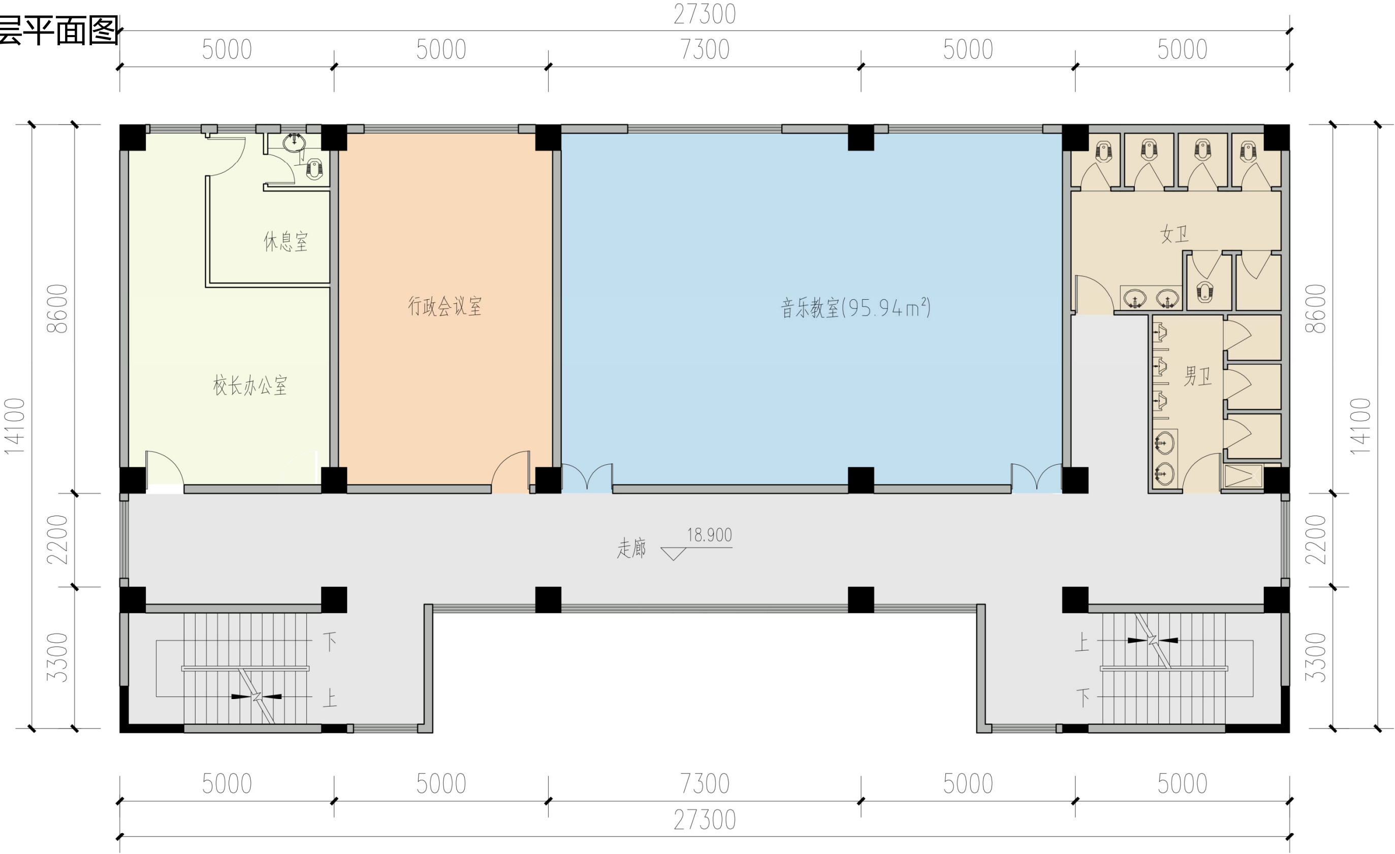
五层平面图
