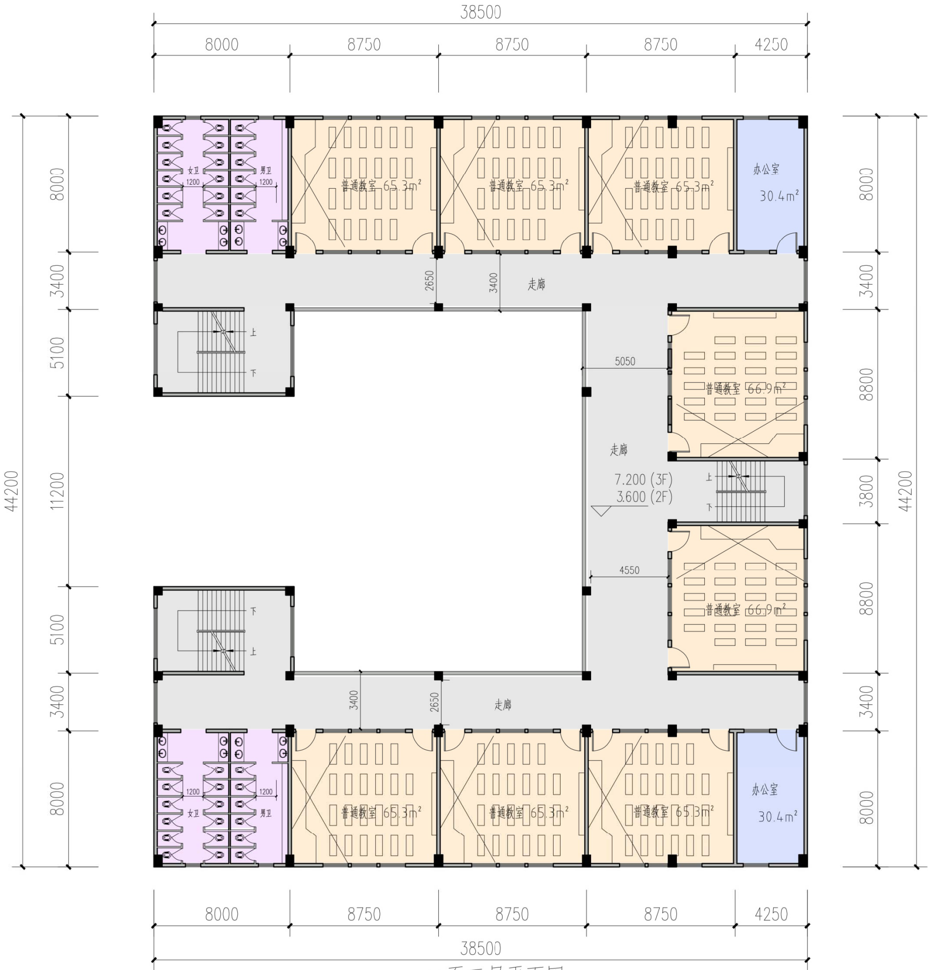
二至三层平面图
