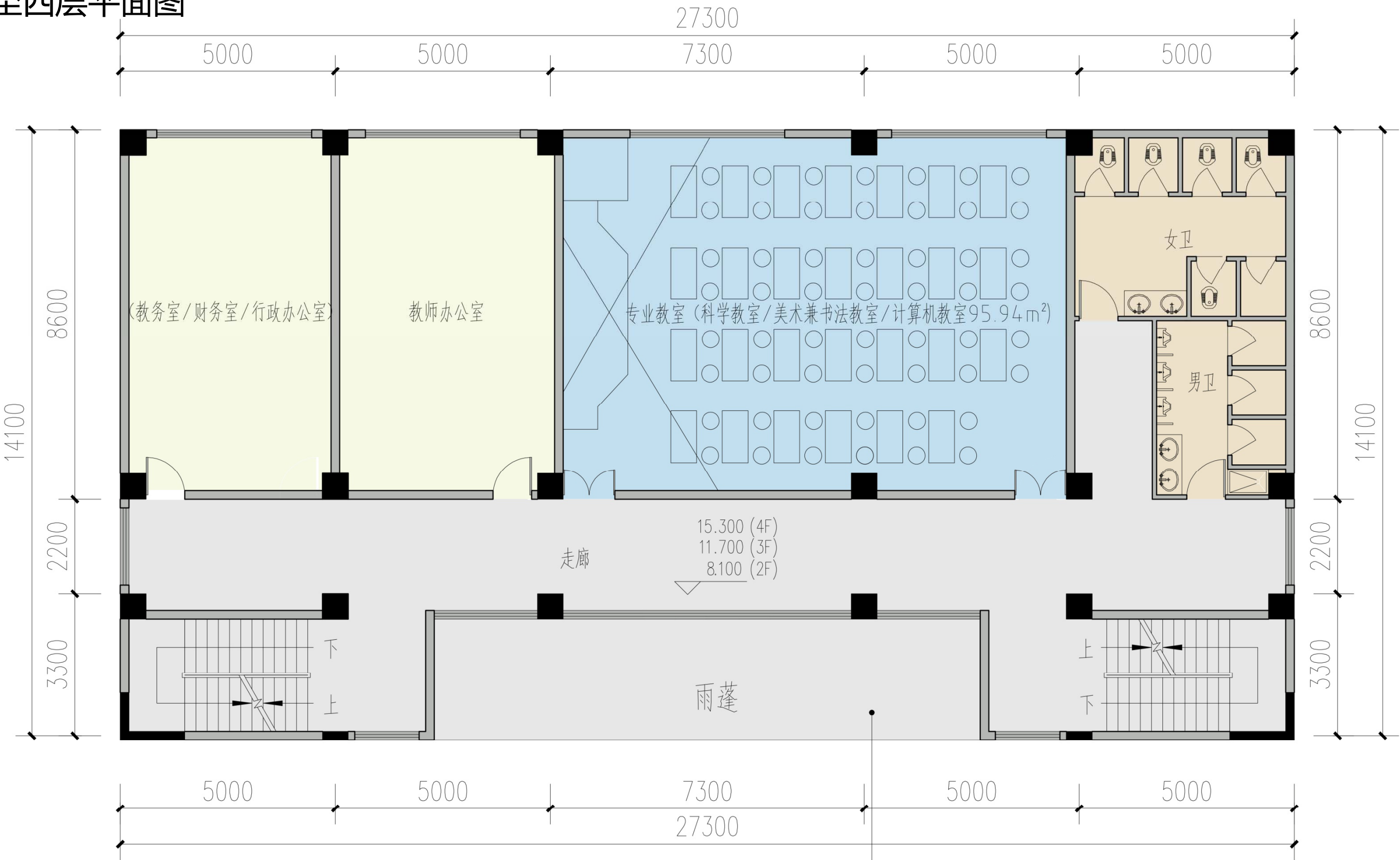
二至四层平面图
