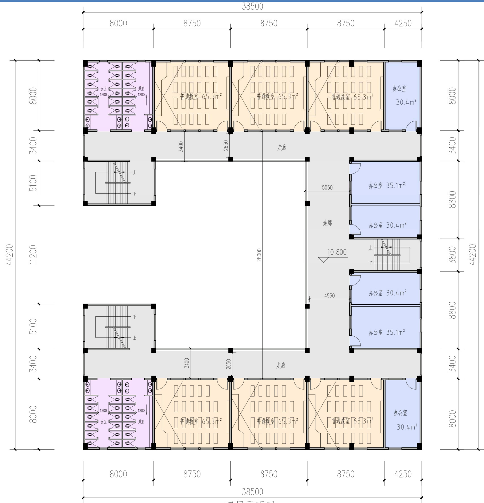
四层平面图 本层建筑面积: 1120.48m²
