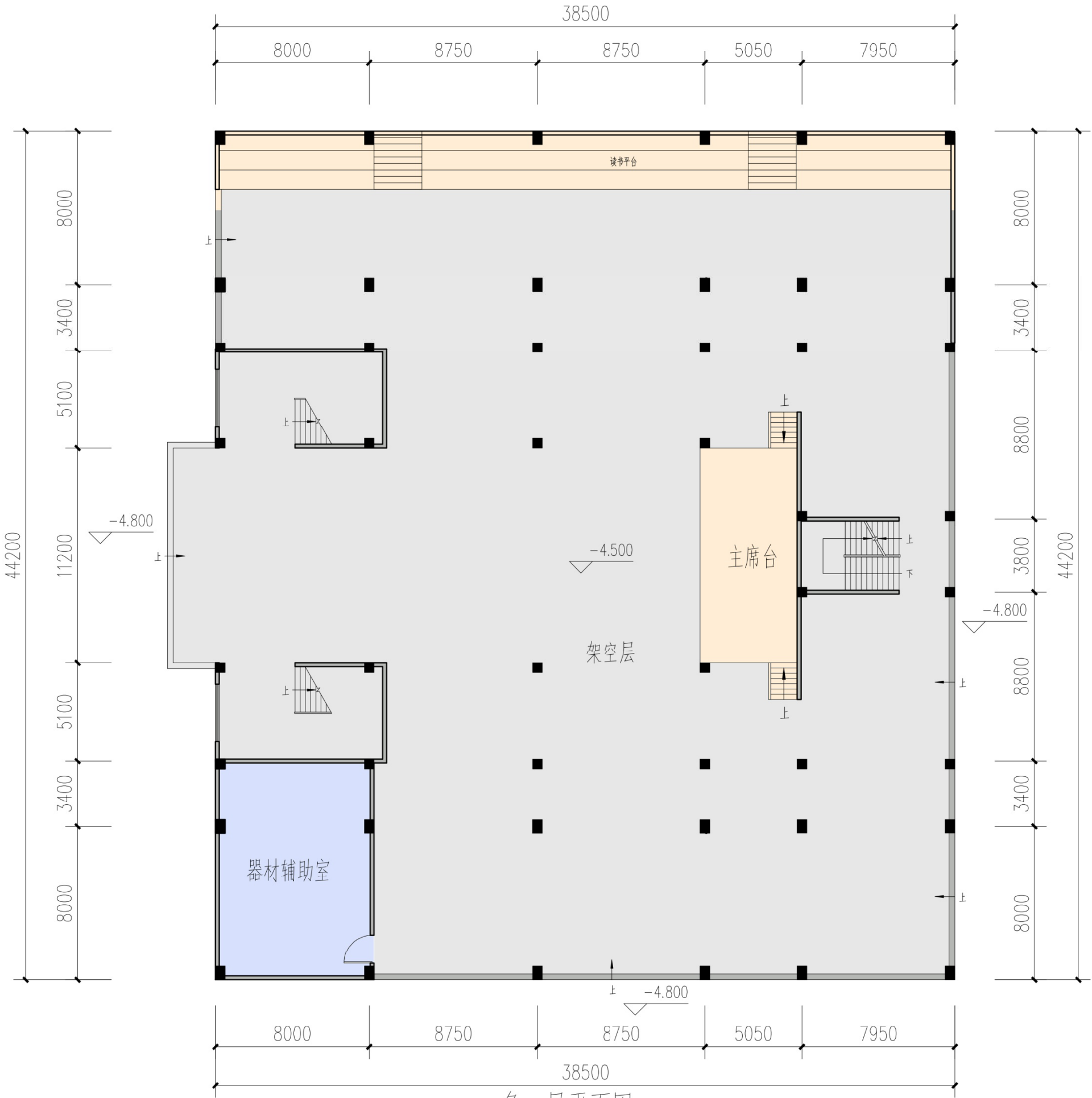
负一层平面图
