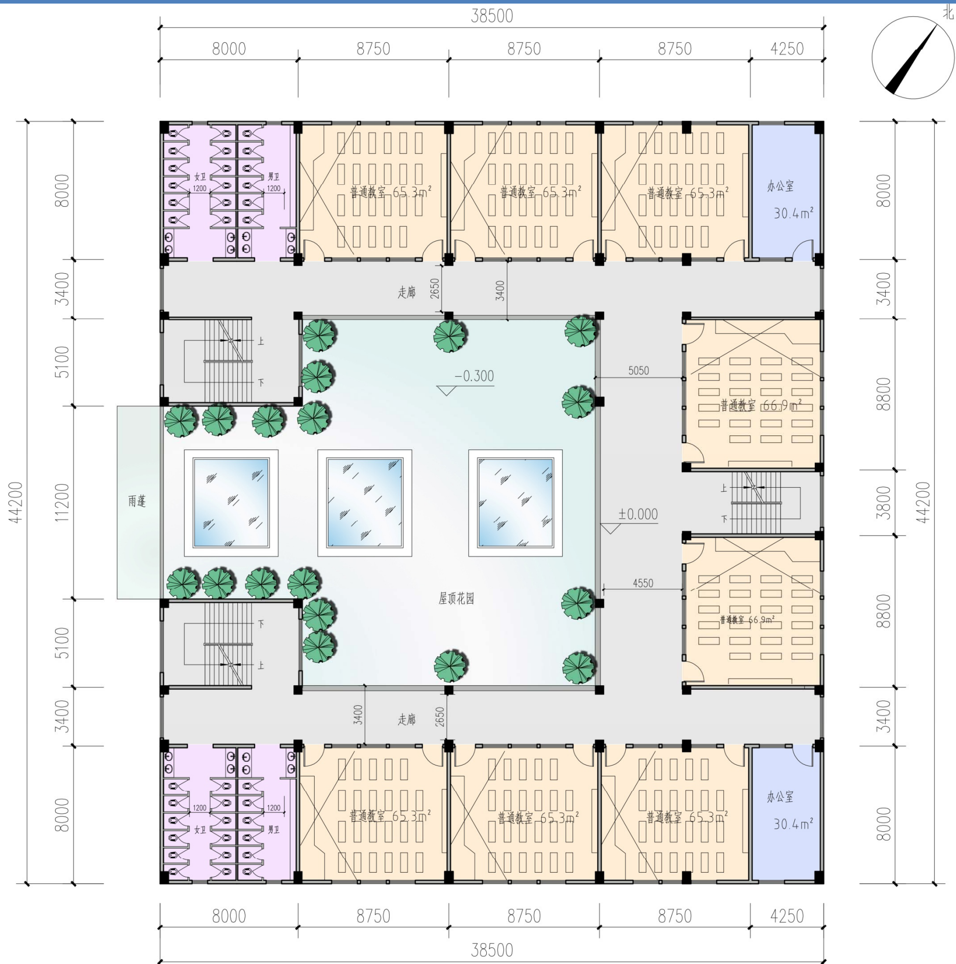
首层平面图
