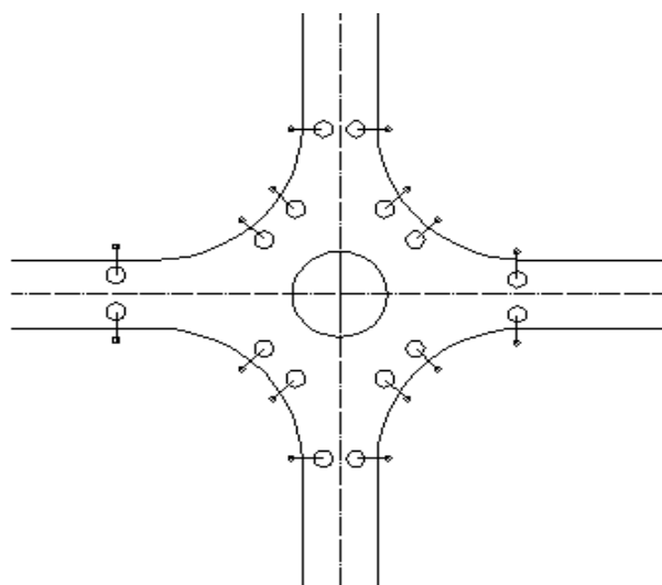
典型布灯方式
