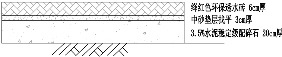
人行道路面结构图 1:10
