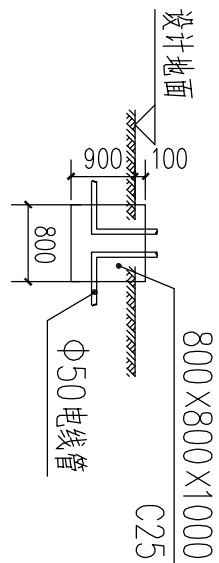
路灯基础图
